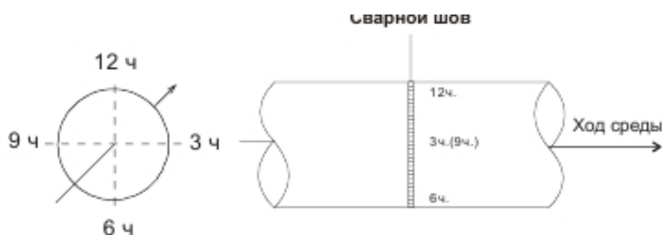
Рисунок 3 - Схема ультразвуковой дефектоскопии сварного шва и околошовной зоны (вид на сечение показан в направлении движения перекачиваемой среды)
